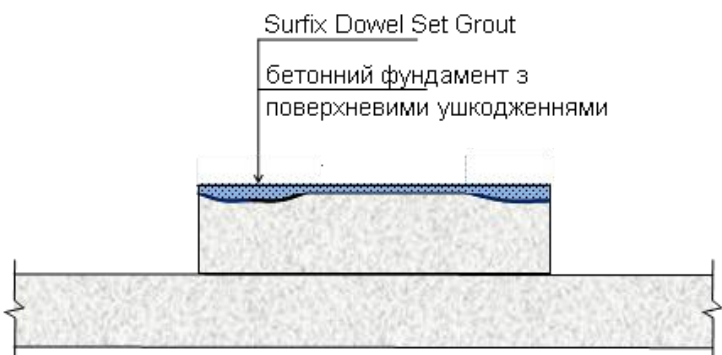
Рисунок П-19. Стандартна схема відновлення бетонного фундаменту з поверхневими ушкодженнями під стаціонарне технологічне устаткування
