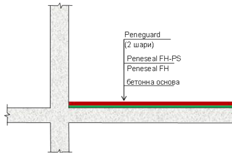
Рисунок I-13-2. Стандартна схема улаштування зносостійких підлогових покриттів для приміщень харчової та фармацевтичної промисловості
