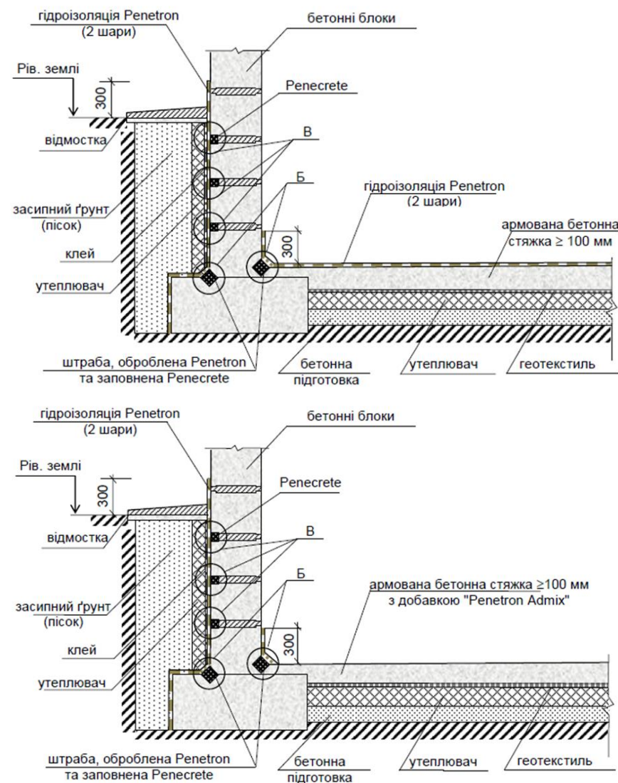
Рисунки II-2-4 і II-2-5. Схеми улаштування зовнішньої і внутрішньої гідроізоляції збірних конструкцій стін та фундаментних плит Примітка: Вузли Б і В див. п. I-5
