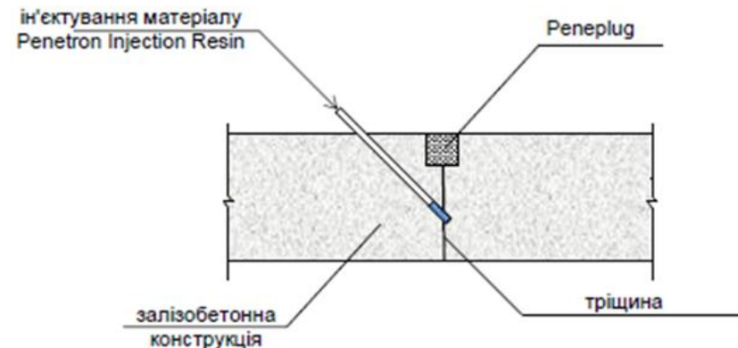
Рисунок I-10-3. Схема улаштування ущільнення обмежено рухомих сухих тріщин
