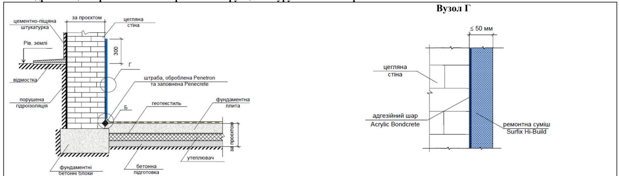
Рисунок П-3-1. Схема улаштування внутрішньої гідроізоляції вертикальних поверхонь конструкцій із мурувальних матеріалів (без капілярного підсмоктування)
