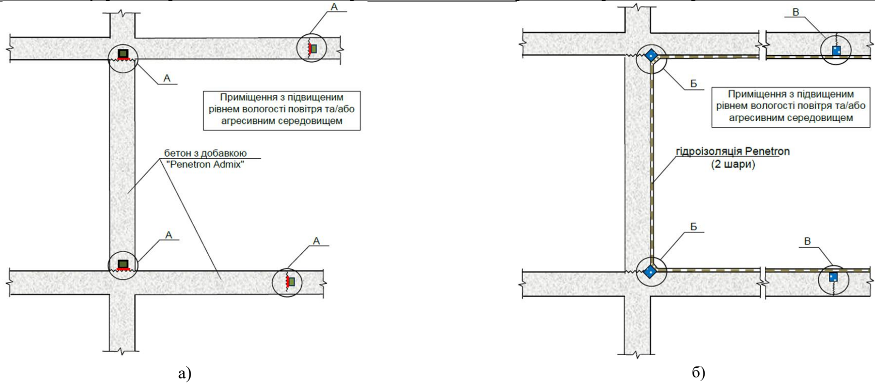
Рисунки I-10-1 і I-10-2. Схеми улаштування гідроізоляції внутрішніх приміщень із застосуванням щільного бетону з добавкою в бетон Penetron Admix (а) та гідроізоляційного матеріалу проникаючої дії Penetron (б)
