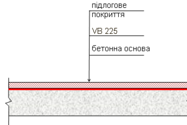
Рисунок I-17-2. Стандартна схема конструкції підлог, що експлуатуються у вологих та/або лужних умовах
