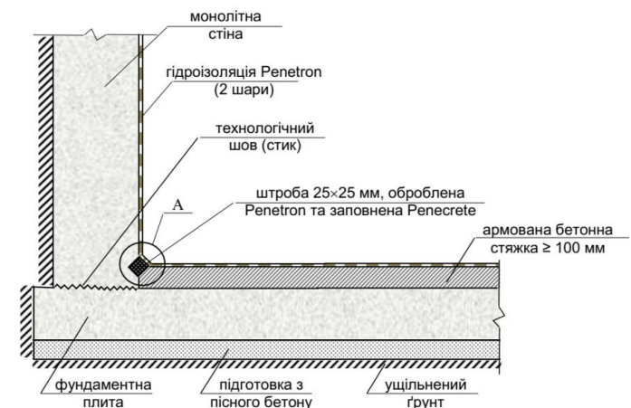
Рисунок 1 Приклад стандартної схеми конструкції із застосуванням Penetron.
