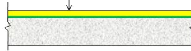
Рисунок I-16. Стандартна схема конструкції самонівелюючих декоративних зносостійких промислових підлог
