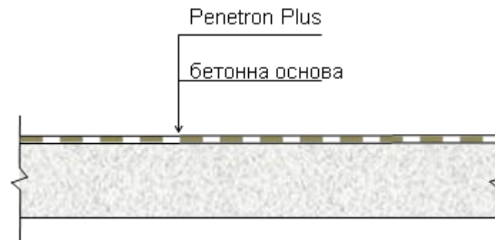
Рисунок I-15-2. Стандартна схема конструкції промислової підлоги з підвищеним рівнем стійкості до ударів та стирання
