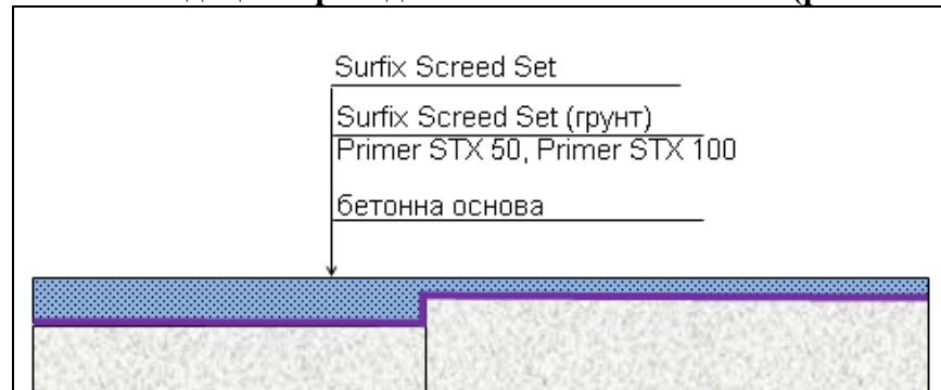
Рисунок П-18. Стандартна схема ліквідація перепадів висотного положення (рівнів чистої підлоги) бетонних підлог суміжних приміщень
