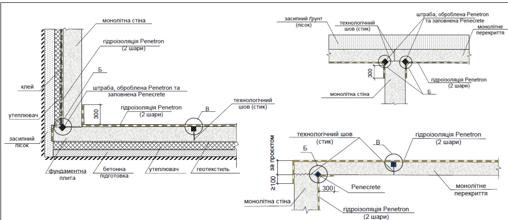
Рисунки П-1-4 і П-1-5. Схеми улаштування внутрішньої і зовнішньої гідроізоляції монолітних стін, фундаментних плит та монолітного перекриття
